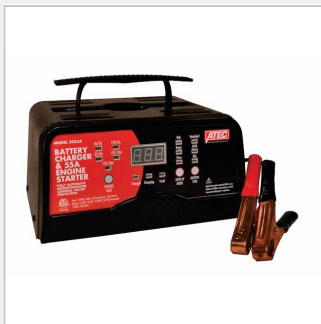
ATEC BATTERY CHARGER, 6/12V 10/2A AUTOMATIC, 50A START/Chargeur à batterie ATEC 6/12V, 10/2A automatique, 50A démarrage Code : ASE / 117 / 3055A
