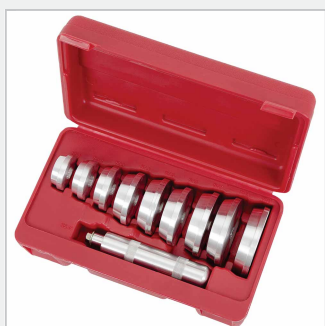
Jeu de 10 pcs mandrins de pose et dépose pour bagues de roulement et joints Code : JET / 790 / H3437
