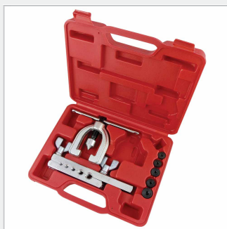
Jeu d'outils à évaser à double recouvrement métrique Code : JET / 790 / H1121
